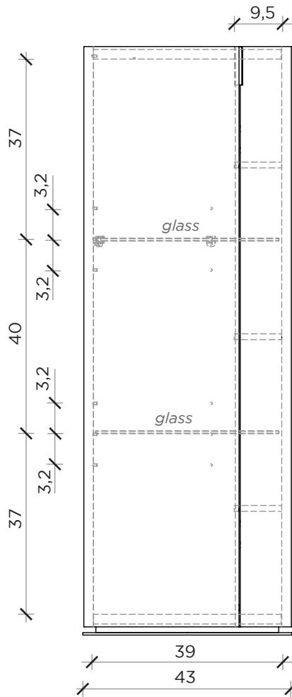
LATO | SIDE
