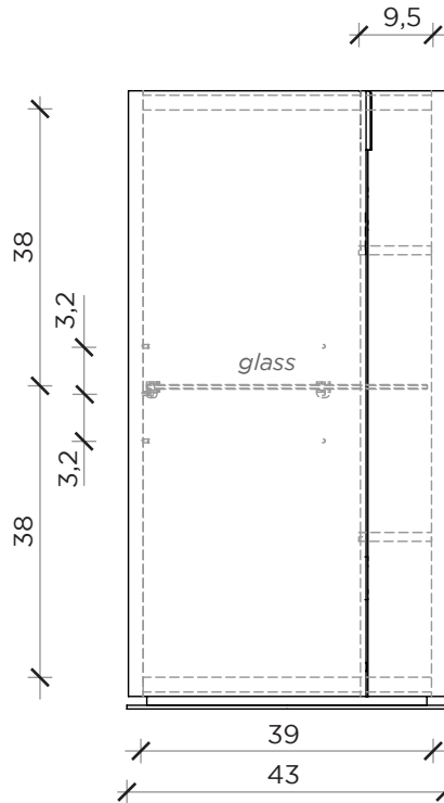
LATO | SIDE
