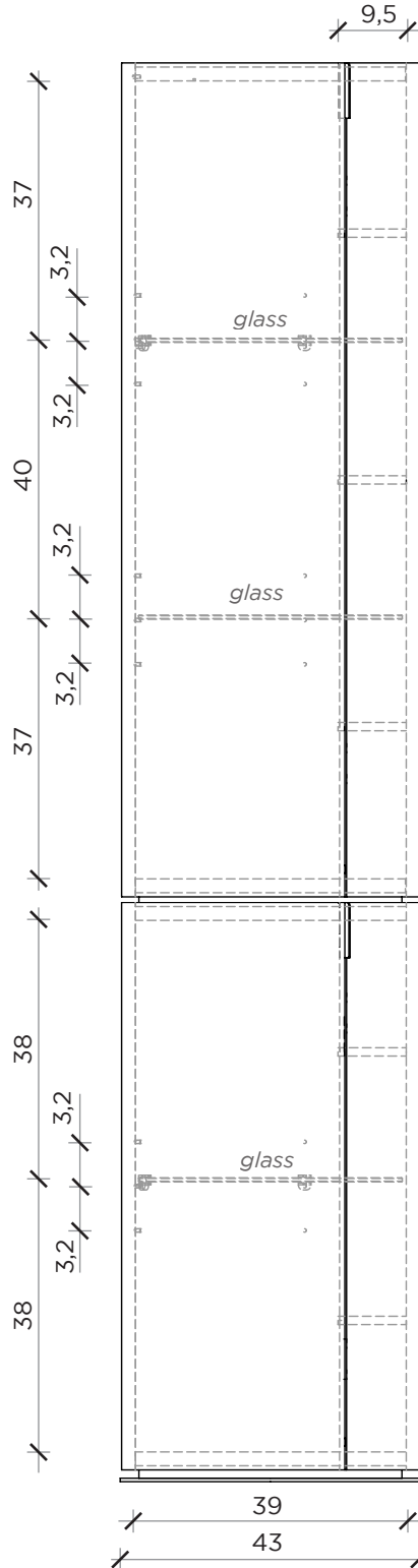
LATO | SIDE
